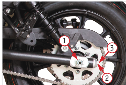
Фото 5.9 Регулировка цепи: 1 - гайка задней оси; 2 - стопорная гайка; 3 - регулировочный болт
