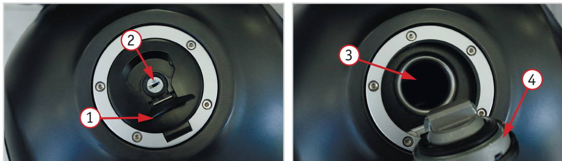
Фото 2.6. Топливный бак: 1 - защитная створка замочной скважины топливного бака; 2 - замочная скважина топливного бака; 3 - горловина топливного бака;
