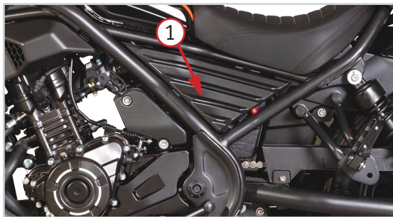
Фото 5.1 Обслуживание воздушного фильтра: 1 - пластиковая накладка
