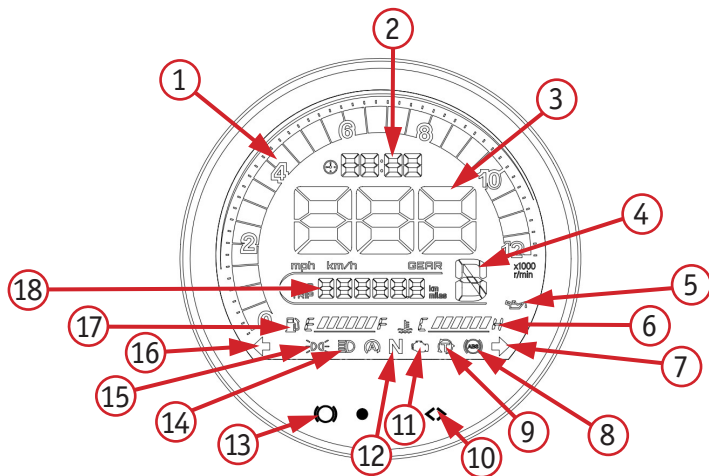
Фото 2.10. Вид приборной панели: 1 – тахометр; 2 – часы; 3 – скорость; 4 – индикатор передачи; 5 – индикатор давления масла; 6 – шкала температуры двигателя; 7 – индикатор правого поворотника; 8 – индикатор ABS; 9 – индикатор системы курсовой устойчивости (TCS); 10 – функциональная кнопка; 11 – индикатор неисправности EFI; 12 – индикатор нейтральной передачи; 13 – кнопка подтверждения; 14 – индикатор дальнего света; 15 – индикатор габаритных огней; 16 – индикатор левого поворотника; 17 – шкала количества топлива; 18 – общий/текущий пробег
