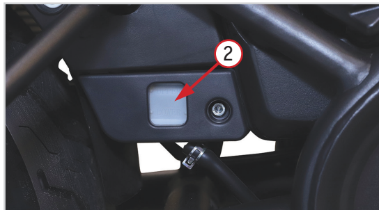
Фото 5.8 Уровень тормозной жидкости переднего и заднего тормозов: 1 – крышка; 2 – отметки минимум и максимум
