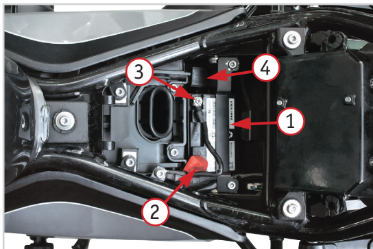
Фото 4.1 Аккумуляторный отсек: 1 – аккумуляторная батарея (АКБ); 2 – клемма «плюс»; 3 – клемма «минус»; 4 – блок предохранителей
