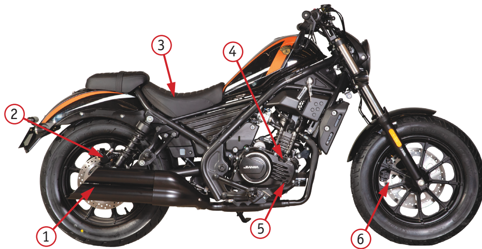
Фото 2.2. Вид справа: 1 – глушитель; 2 – задние дисковые тормоза; 3 – сиденье; 4 – заливная горловина для масла; 5 – педаль заднего тормоза; 6 – передние дисковые тормоза
