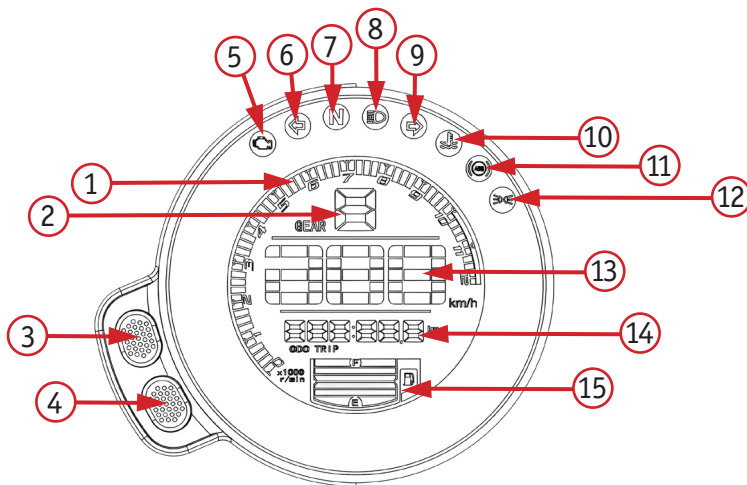
Фото 2.10. Вид приборной панели: 1 – тахометр; 2 – индикатор передачи; 3 – кнопка «Вверх»; 4 – кнопка «Вниз»; 5 – индикатор неисправности EFI; 6 – индикатор левого поворотника; 7 – индикатор нейтральной передачи; 8 – индикатор дальнего света; 9 – индикатор правого поворотника; 10 – индикатор перегрева двигателя; 11 – индикатор ABS; 12 – индикатор габаритных огней; 13 – скорость; 14 – общий/текущий пробег; 15 – количество топлива
