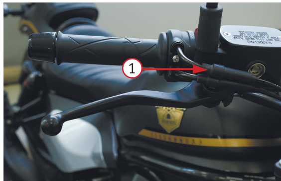
Фото 3. Регулировка троса газа: 1 – защитный колпачок
