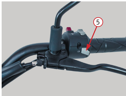
Фото 2.4 Левый комбинированный переключатель: 1 – переключатель режима света фары (дальний свет/ ближний свет); 2 – клавиша указателей поворота; 3 – кнопка звукового сигнала; 4 – кнопка аварийной сигнализации; 5 – кнопка включения дальнего света при обгоне
