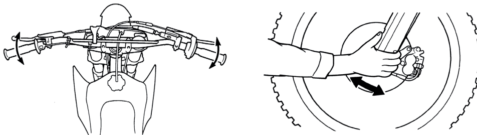
Рисунок 4. Проверка рулевой колонки
