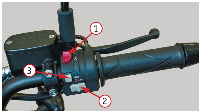
Фото 2.5. Правый комбинированный переключатель: 1 – кнопка электростартера; 2 – переключатель освещения; 3 – кнопка «MODE»
