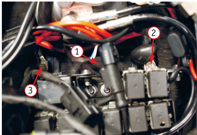
Фото 4. Аккумуляторный отсек: 1 – аккумуляторная батарея (АКБ); 2 – клемма «плюс»; 3 – клемма «минус»
