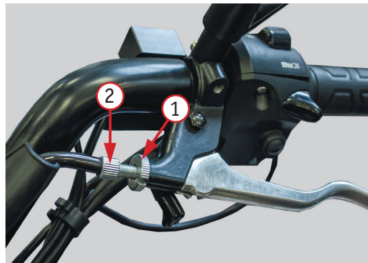
Фото 2.11. Регулировка сцепления: 1 – стопорная гайка; 2 – регулировочный винт
