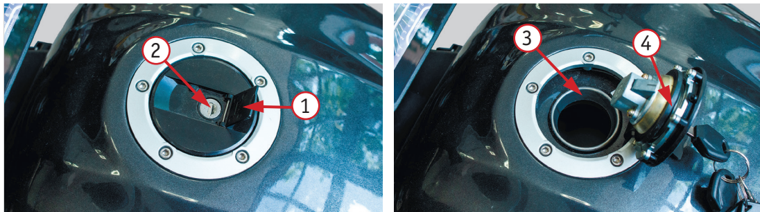
Фото 2.6. Топливный бак: 1 - защитная створка замочной скважины топливного бака; 2 - замочная скважина топливного бака; 3 - горловина топливного бака; 4 - крышка топливного бака в открытом виде
