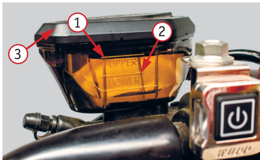
Фото 5.7.1. Уровень тормозной жидкости переднего тормоза: 1 – максимум; 2 – минимум; 3 – крышка
