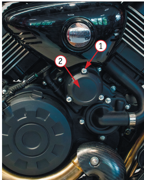
Фото 5.6. Замена масляного фильтра: 1 – винты крышки; 2 – крышка масляного фильтра
