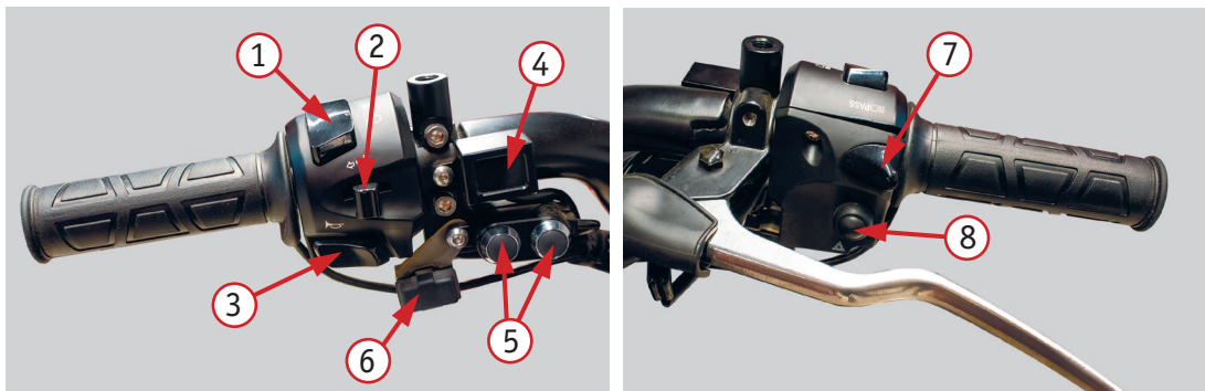
Фото 2.4. Левый комбинированный переключатель: 1 – кнопка переключения режима света фары (дальний свет/ближний свет); 2 – переключатель указателей поворота; 3 – кнопка звукового сигнала; 4 – индикатор высоты пневматической подвески; 5 – кнопки уменьшения/увеличения высоты пневматической подвески; 6 – порт USB; 7 – кнопка включения дальнего света при обгоне; 8 – кнопка аварийной сигнализации
