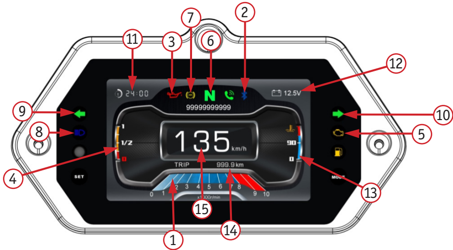
Фото 2.10. Вид приборной панели: 1 – тахометр; 2 – индикатор подключения Bluetooth; 3 – индикатор пониженного давления масла; 4 – количество топлива; 5 – индикатор неисправности EFI; 6 – индикатор передачи; 7 – индикатор ABS; 8 – индикатор дальнего света; 9 – индикатор левого поворотника; 10 – индикатор правого поворотника; 11 – время; 12 – напряжение батареи; 13 – температура двигателя; 14 – общий пробег; 15 – скорость
