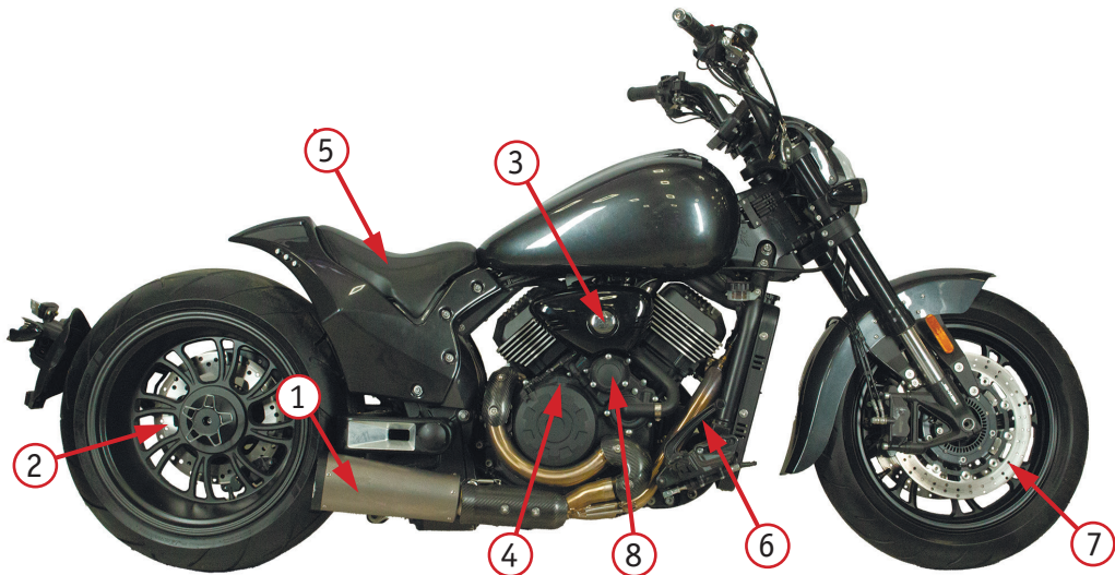
Фото 2.2. Вид справа: 1 – глушитель; 2 – задние дисковые тормоза; 3 – замок зажигания; 4 – заливная горловина для масла; 5 – сиденье; 6 – рычаг заднего тормоза; 7 – передние дисковые тормоза; 8 – крышка масляного фильтра
