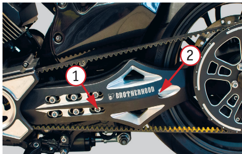
Фото 5.8. Регулировка ремня: 1 - стопорный болт; 2 - регулировочный болт
