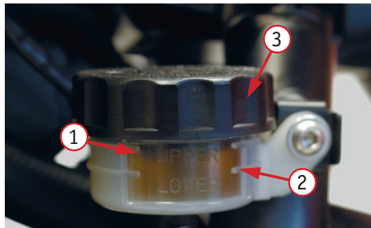
Фото 5.7.2. Уровень тормозной жидкости заднего тормоза: 1 – максимум; 2 – минимум; 3 – крышка
