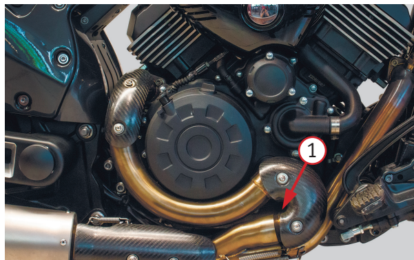
Фото 5.3. Окно для контроля уровня масла – 1 (находится за выхлопной трубой)
