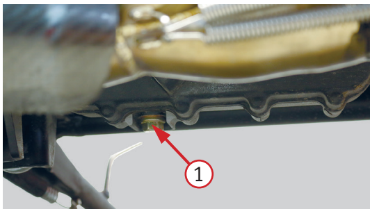
Фото 5.5. Болт слива масла - 1
