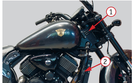
Фото 1.2. Идентификационный код транспортного средства (VIN) 1 и идентификационная табличка 2 расположены на правой стороне передней части мотоцикла
